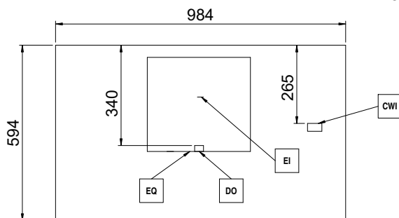
Planta
